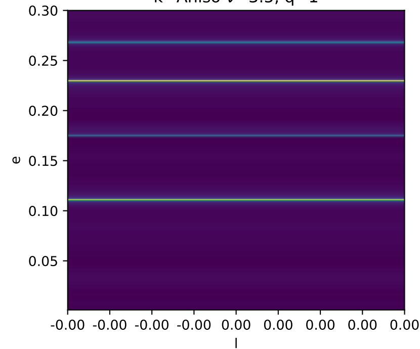
k=Aniso \nu=3.5 , q=1
